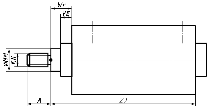
Рисунок 1 — Основные размеры
