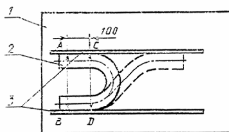
1 — контрольная плита; 2 — изделие; 3 — поверочные линейки Черт. 16
