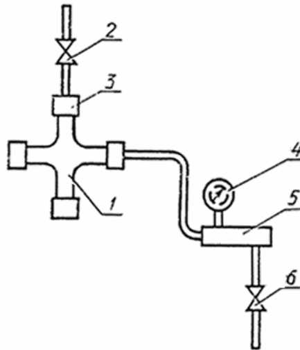
1 — изделие; 2 — кран для выпуска воздуха; 3 — заглушки; 4 — манометр; 5 — насос; 6 — кран для подачи воды
