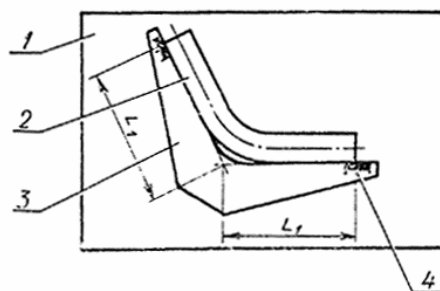
1 — контрольная плита; 2 — изделие; 3 — шаблон; 4 — поле допуска Черт. 15
