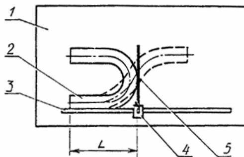
1 — контрольная плита; 2 — изделие; 3 — контрольная линейка; 4 — ползун; 5 — упор Черт. 14
