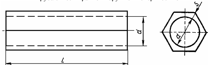
Труба с шестигранной наружной поверхностью
