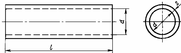
Труба с цилиндрической наружной поверхностью
